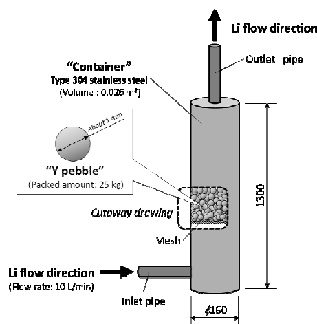
Trampa de Y prevista para ELTL (EVEDA Lithium Test Loop), Oarai, Japón
