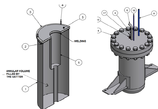
Trampa experimental de nitrógeno de LIFUS 6 (ENEA) (19 l de litio, 8.2 Kg de Ti (getter), 550 y 600°C)
