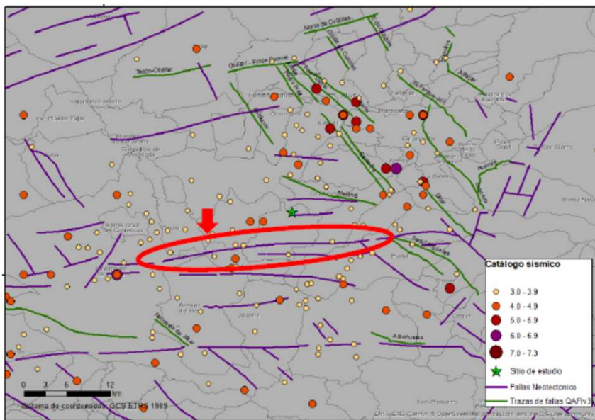
Localización de la Falla Sur de Escúzar
